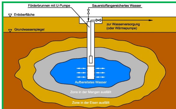
Wirkbereich - Unterirdische Enteisenung
